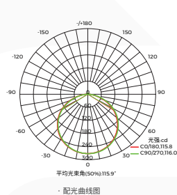
· 配光曲线图
